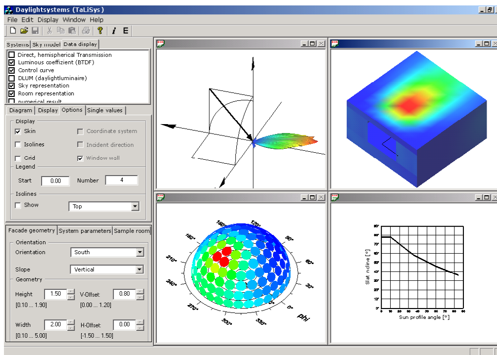
Abbildung 4 Expertenmodus des Planungswerkzeuges: BTDF(links oben); Himmelsleuchtdichteverteilung (links unten); Raumbelichtung durch das ausgewählte System (rechts oben); Steuerkennlinie (rechts unten)
