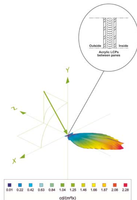
Abbildung 1 Darstellung der räumlichen Verteilung des Leuchtdichtekoeffizienten (sog. Bidirectional Transmission Distribution Function: BTDF) für ein Lichtlenkglas bei einer einfallseitigen Beleuchtung unter einem Höhenwinkel von 48°.
