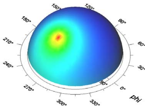
Abbildung 2 Darstellung einer exemplarischen Himmelsleuchtdichteverteilung des klaren Himmels.
