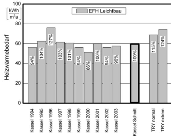
Abbildung 5 Spezifischer jährlicher Heizwärmebedarf Einfamilienhaus Leichtbau
